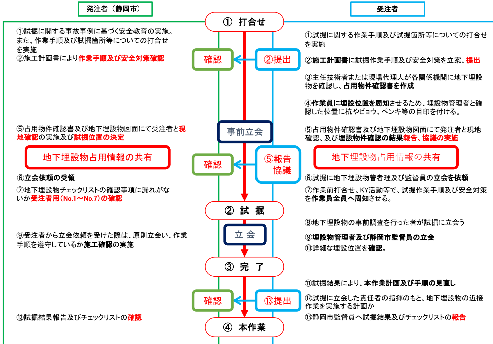
地下埋設物事故防止対策フロー図
