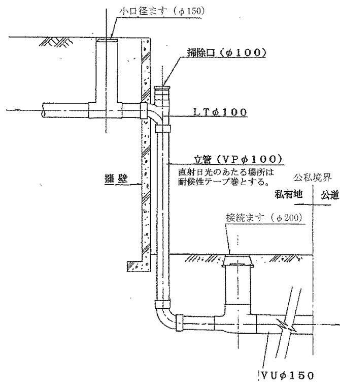
図Ⅲ-17-B 敷地内に擁壁がある場合の例
