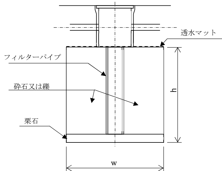
図Ⅲ－８－Ａ 浸透ます構造図
