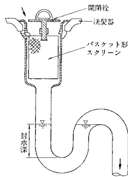
図Ⅱ-14 ヘア阻集器の例
