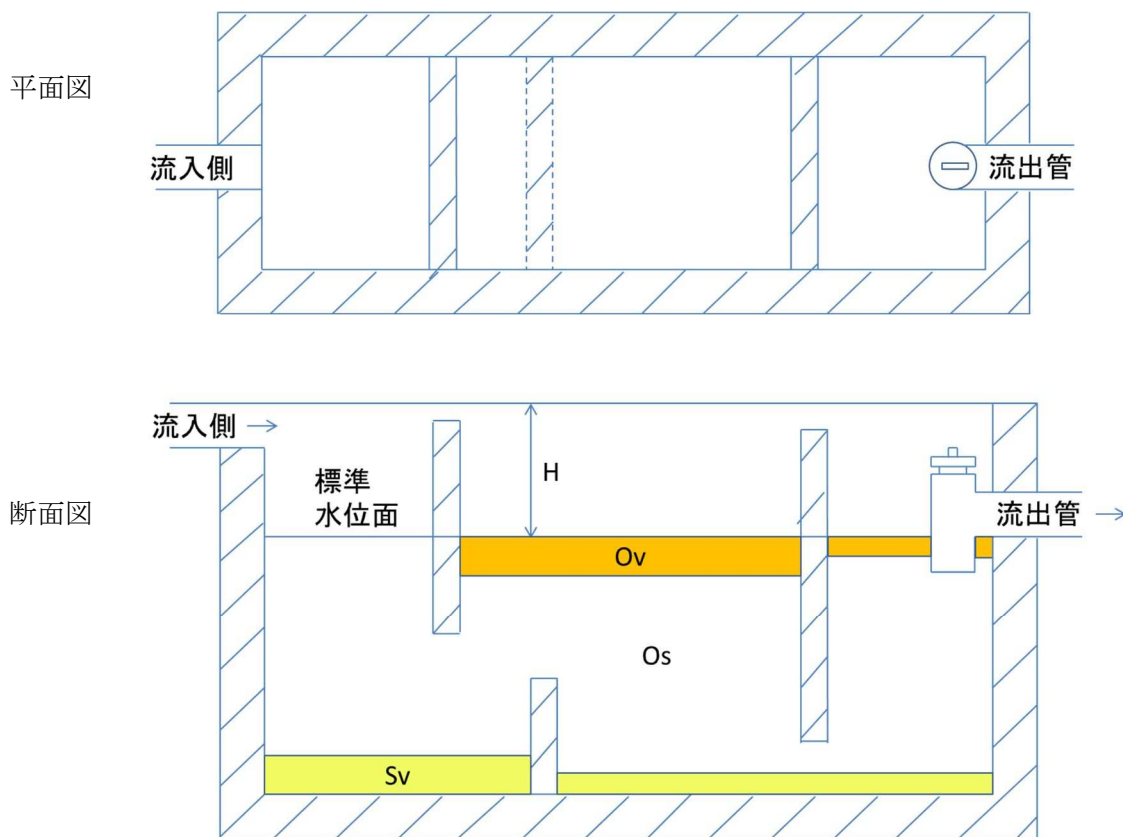
図Ⅶ-2 3槽式オイル阻集器の仕様例
