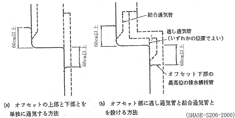
図Ⅱ-22 45^\circ を超えるオフセット部の通気方法
