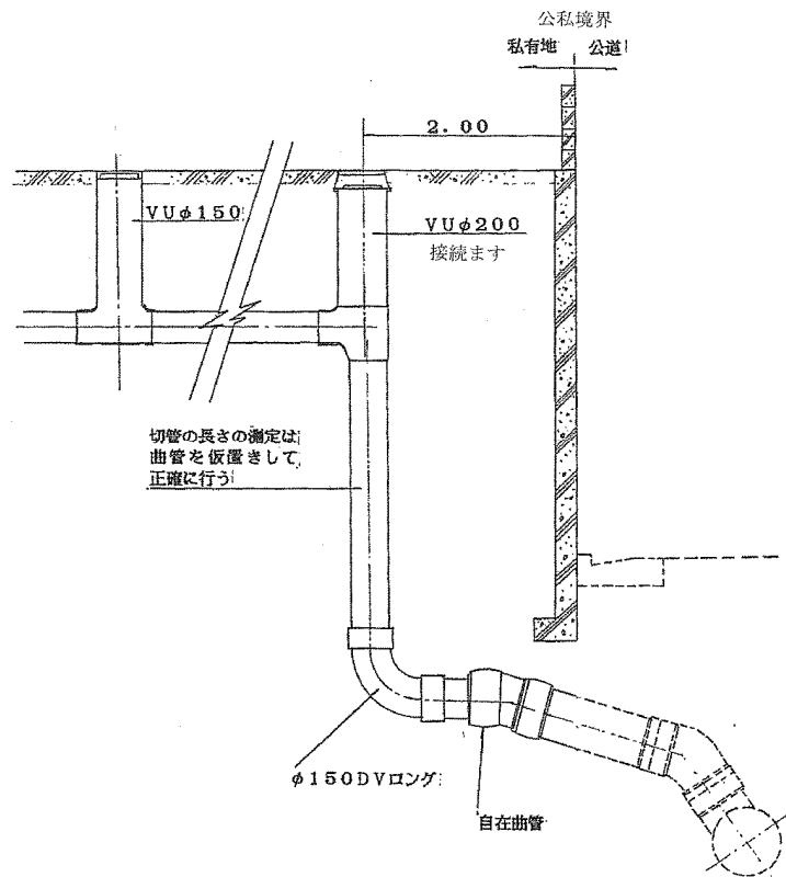
図Ⅲ-17-A 公私境界で上流と下流に著しく落差があるドロップ管の例
