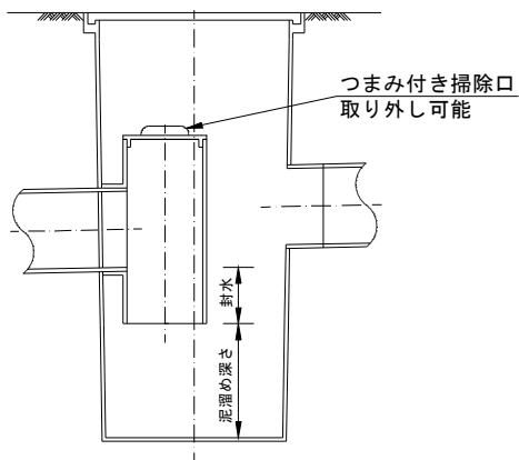
図Ⅲ－12 防臭ます
