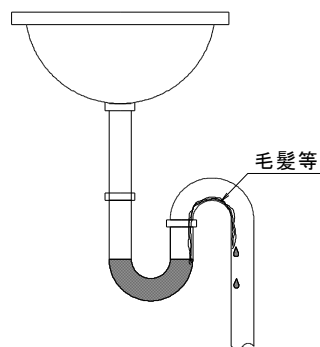
図Ⅱ－７ 毛管現象
