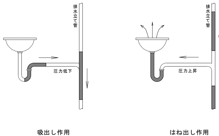
図Ⅱ－６ 吸出し作用とはね出し作用
