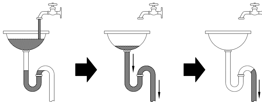
図Ⅱ－５ 自己サイホン作用
