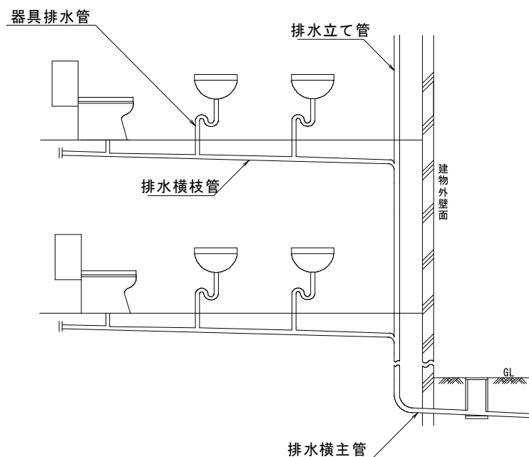
図 II - 1 排水管の種類
