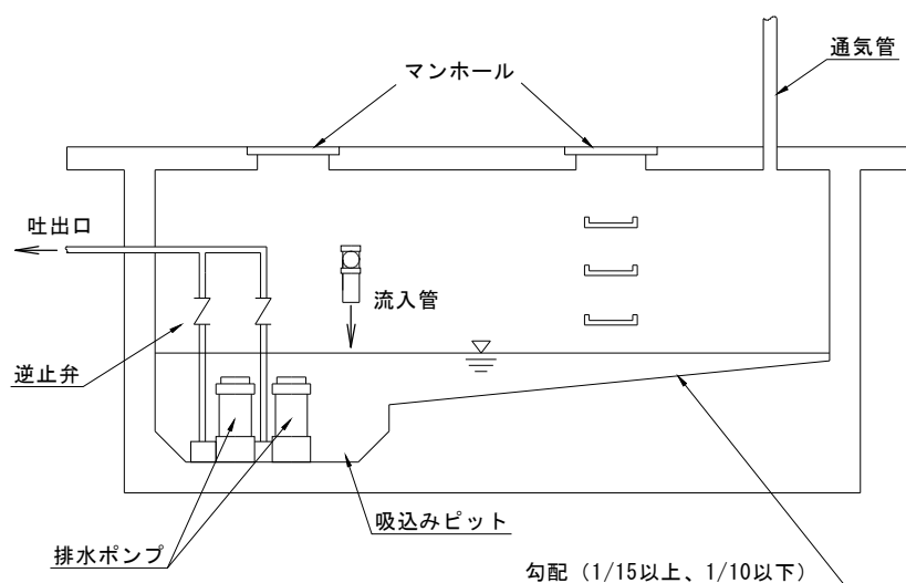
図 II -17 排水槽の構造
