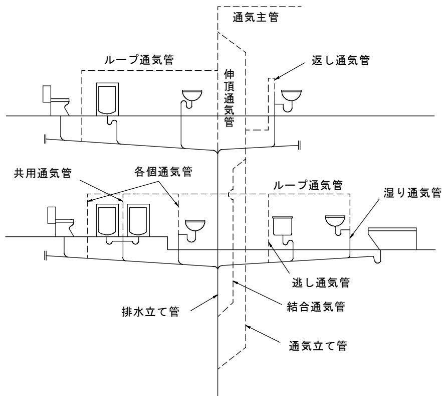
図Ⅱ-18 通気管の種類
