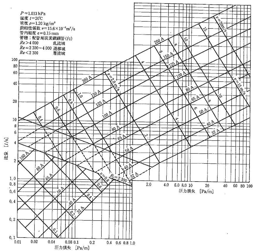
図 X-12 通気管抵抗線図
