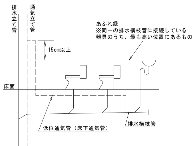
図Ⅱ-21 条件付きで認められる低位通気配管の例
