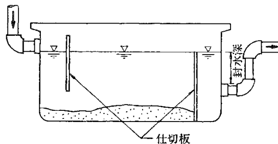
図Ⅱ-13 サンド阻集器の例
