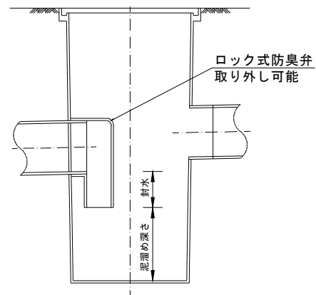
図Ⅲ－12 防臭ます
