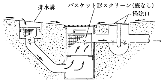
図Ⅱ-15 ランドリー阻集器の例
