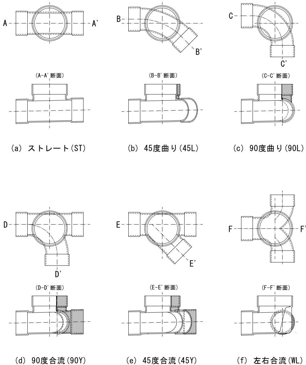
図Ⅲ－11 インバートます（樹脂性）[参考図]
