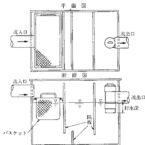
図Ⅱ-11 グリース阻集器の例
