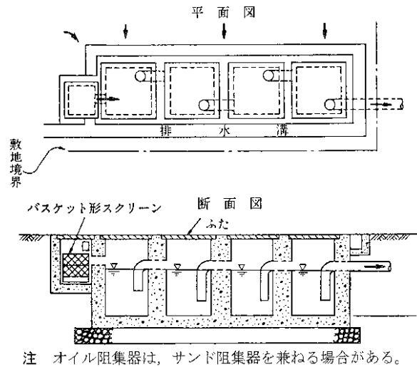
図Ⅱ-12 オイル阻集器の例
