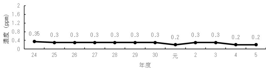
[図 3-16] 一酸化炭素濃度年平均値の経年変化
