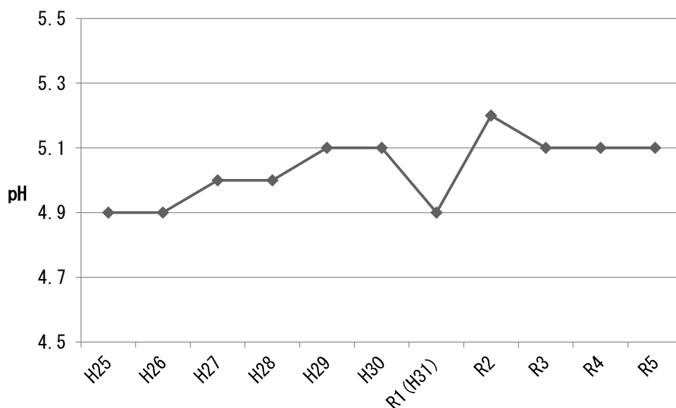
[図 3 - 21] pH の年平均値の推移（平成 25 年度から令和 5 年度）
