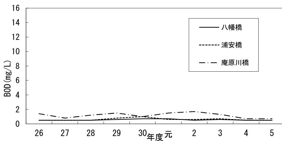
[図 3 - 26] 河川 BOD 環境基準 75%水質値の推移 (その 4)
