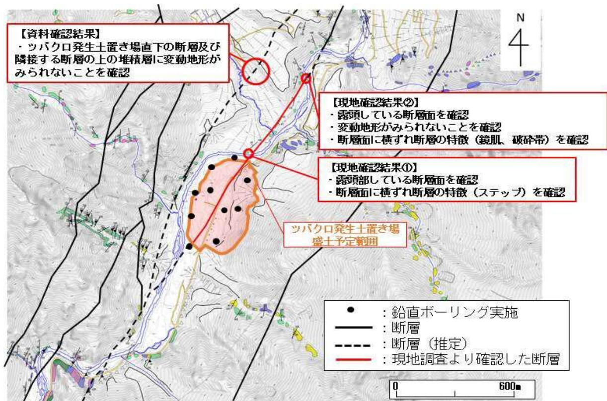
図 30 ツバクロ発生土置き場周辺の調査結果
