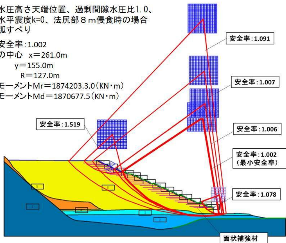
図 1 4 土石流により法尻が侵食された場合の円弧すべり検討結果（補強後）
