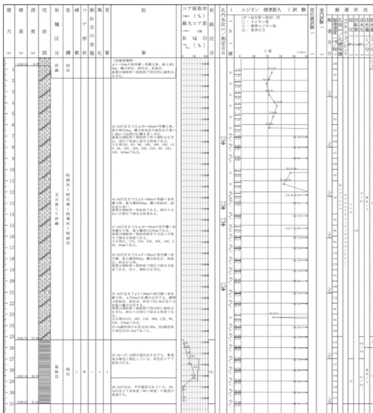
図 40 ツバクロ発生土置き場ボーリング柱状図 (H27 ツバクロ)
