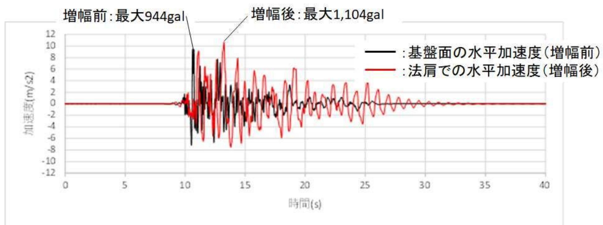
図 2 4 レベル2地震動解析結果
