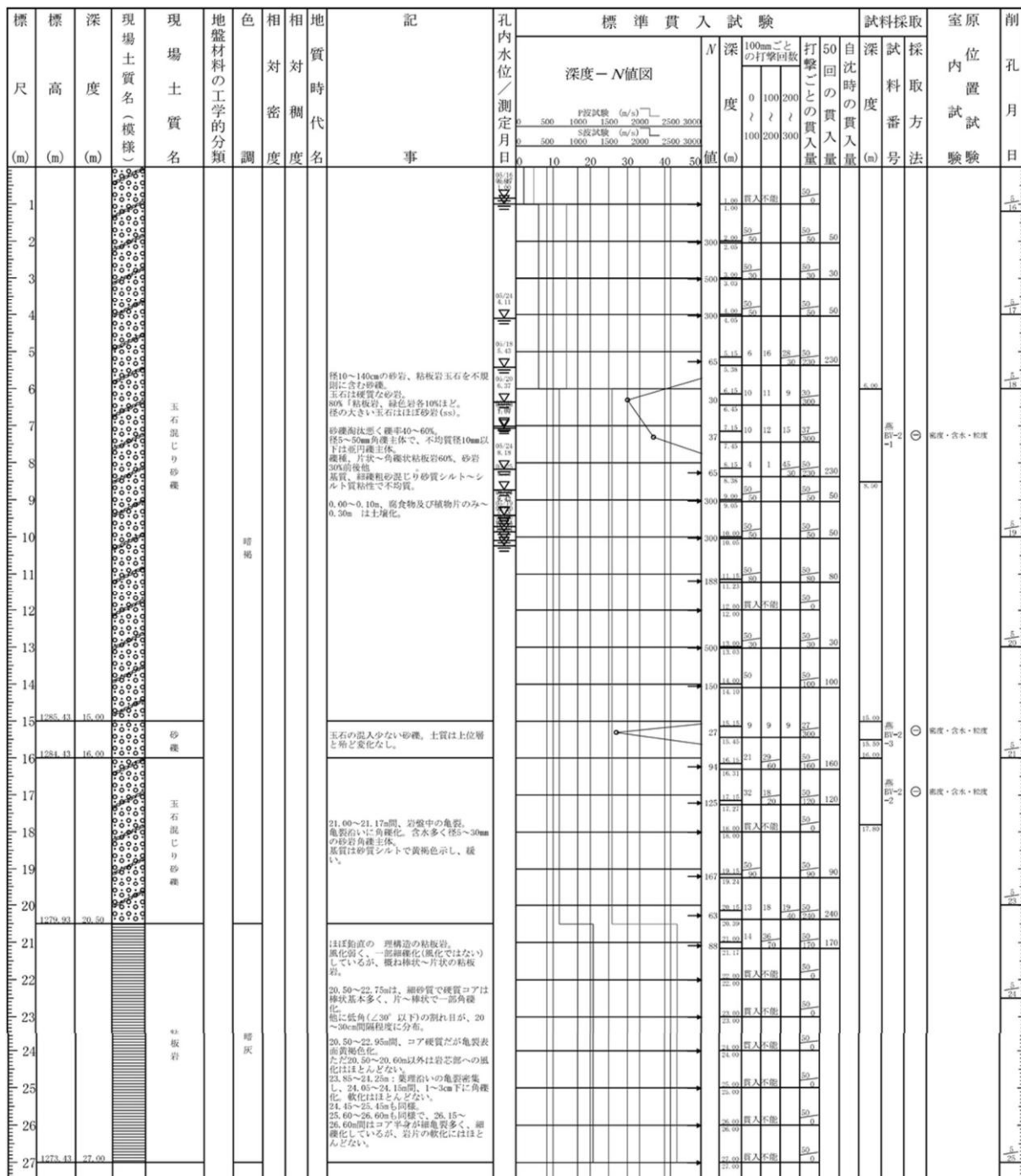
図 45 ツバクロ発生土置き場ボーリング柱状図(燕B V-2)
