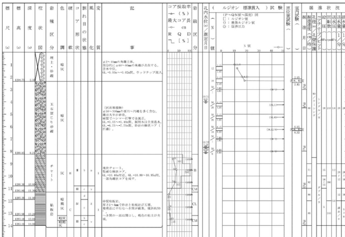
図 39 ツバクロ発生土置き場ボーリング柱状図 (H25 ツバクロ)
