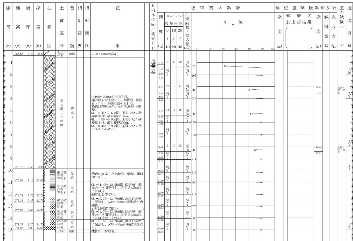
図 4 3 ツバクロ発生土置き場ボーリング柱状図 (燕BV-C)
