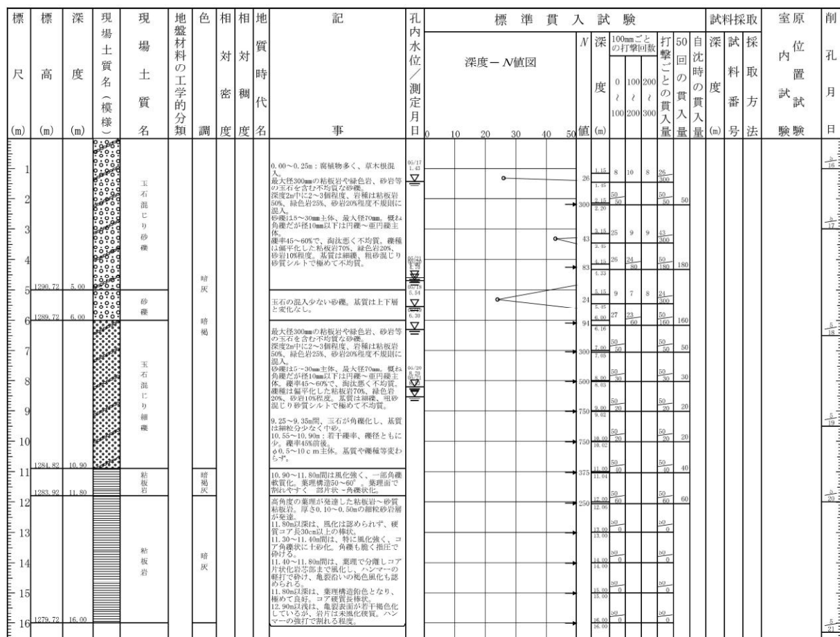
図 46 ツバクロ発生土置き場ボーリング柱状図 (燕BV-3)
