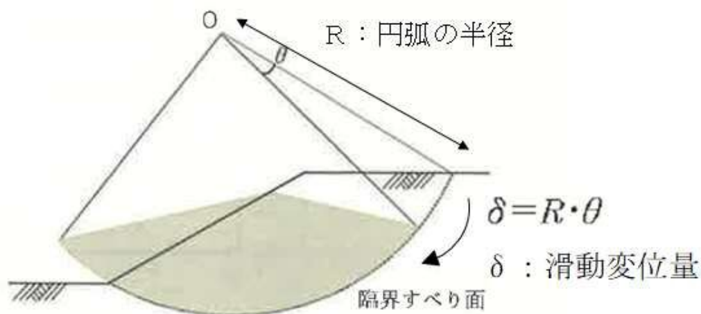
図 25 ニューマーク法の概念図
