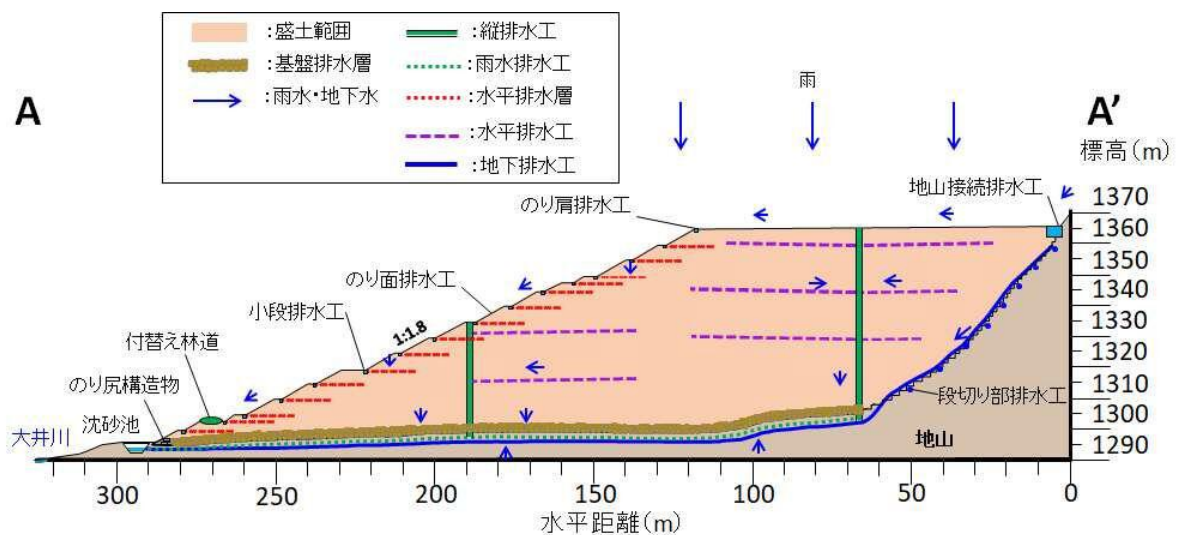
図 3 3 排水設備計画断面図
