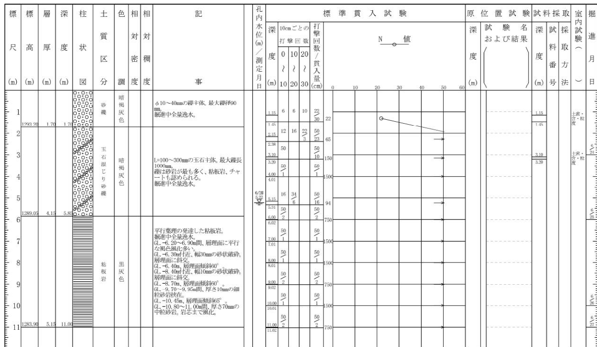
図 4 2 ツバクロ発生土置き場ボーリング柱状図 (燕BV-B)
