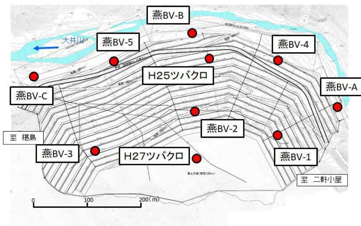
図 ３ ８ ツバクロ発生土置き場ボーリング位置図
