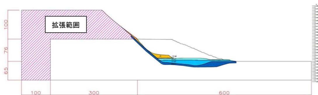
図 2 2 FEM解析に用いたモデル
