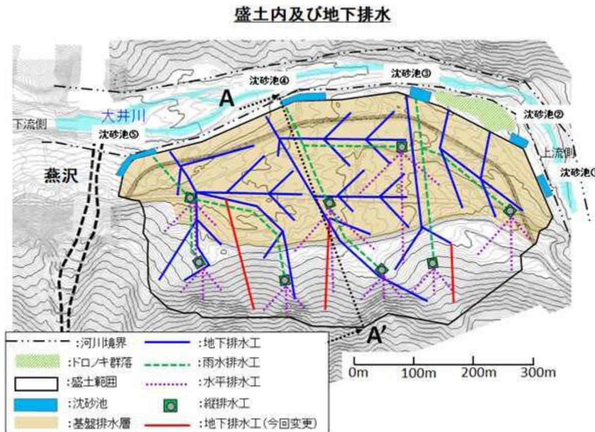
図 3 2 盛土内排水及び地下排水計画図
