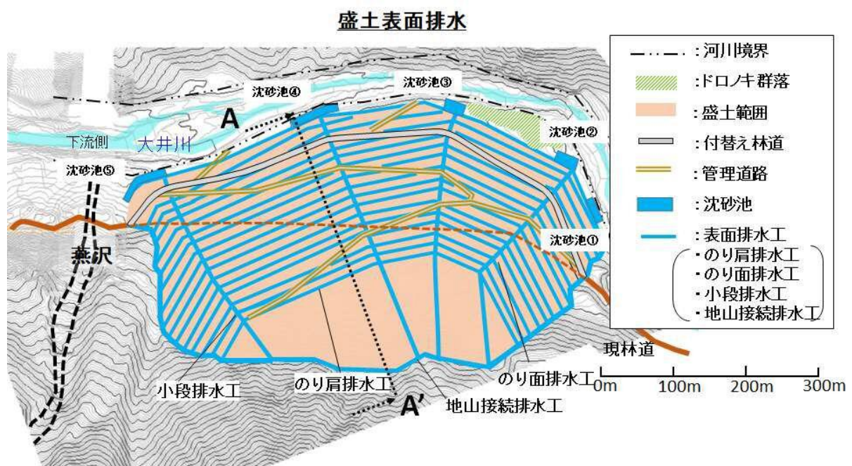
図 3 1 排水設備計画（盛土表面）
