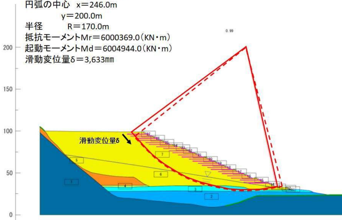
図 26 ニューマーク法による変位量計算結果 (変位量約3.6m)
