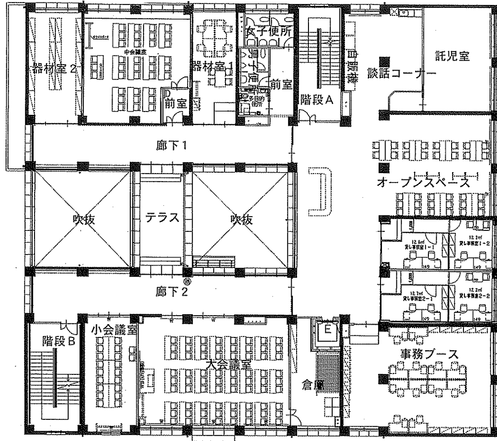
2階 平面図
