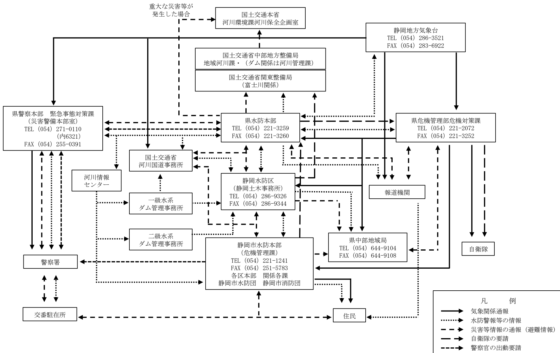
水防時における通信連絡基本系統図
