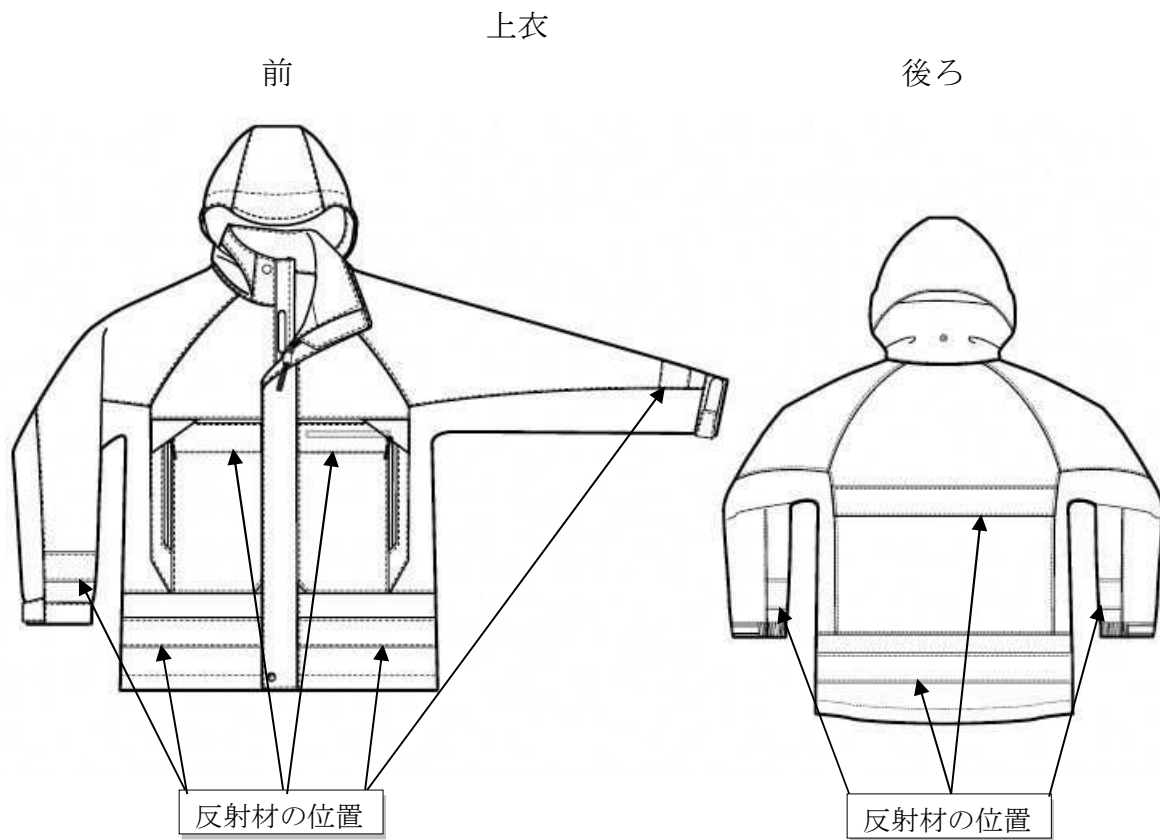
概要図 1
