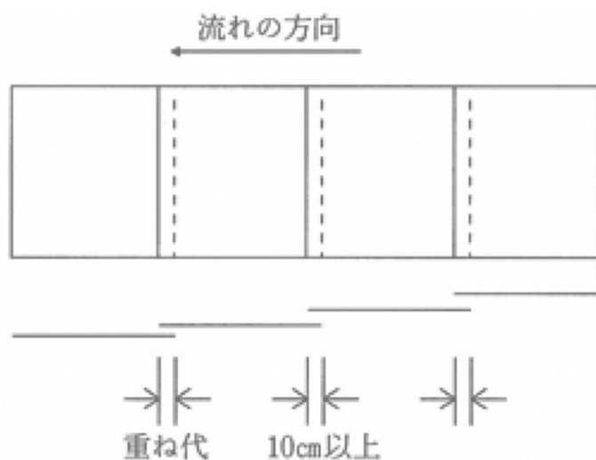
図1-1 吸出し防止シートの重ね代
