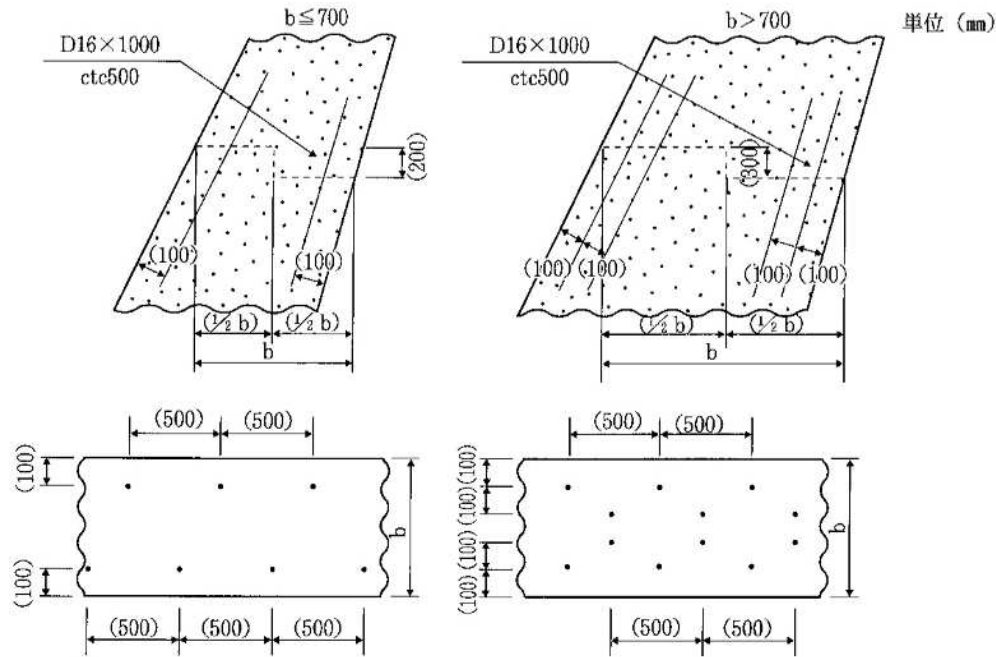
图 3-3 (水平打継目)
