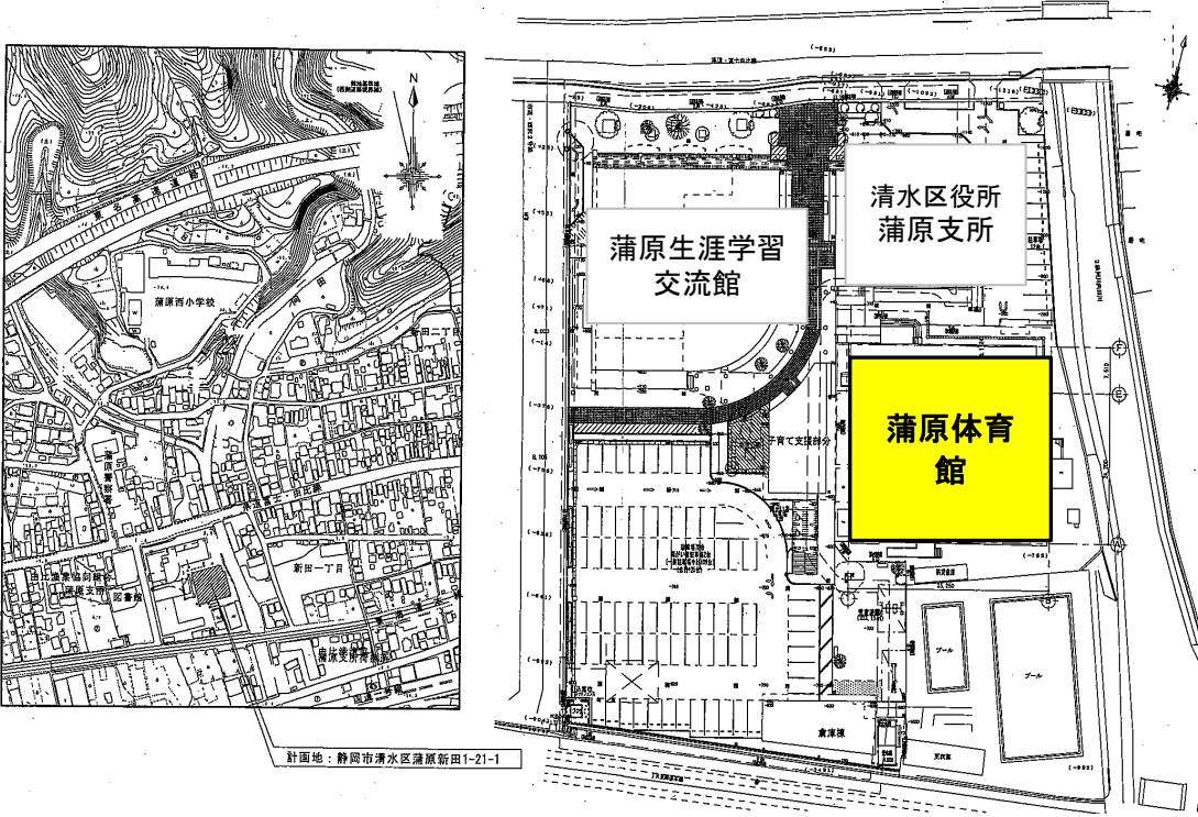
配置図 S=1:400
