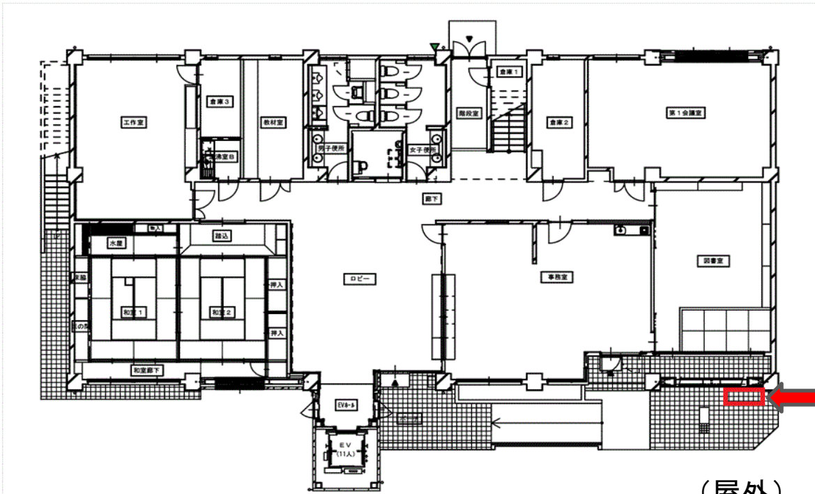
折戸生涯学習交流館 1階平面図
