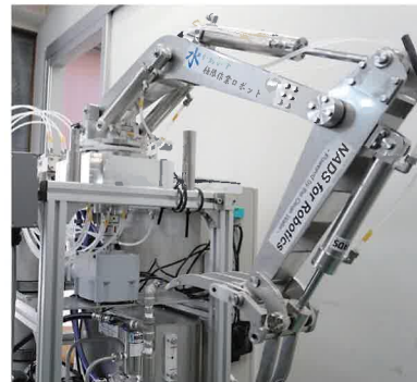
▲水中ロボット(アーム部)
