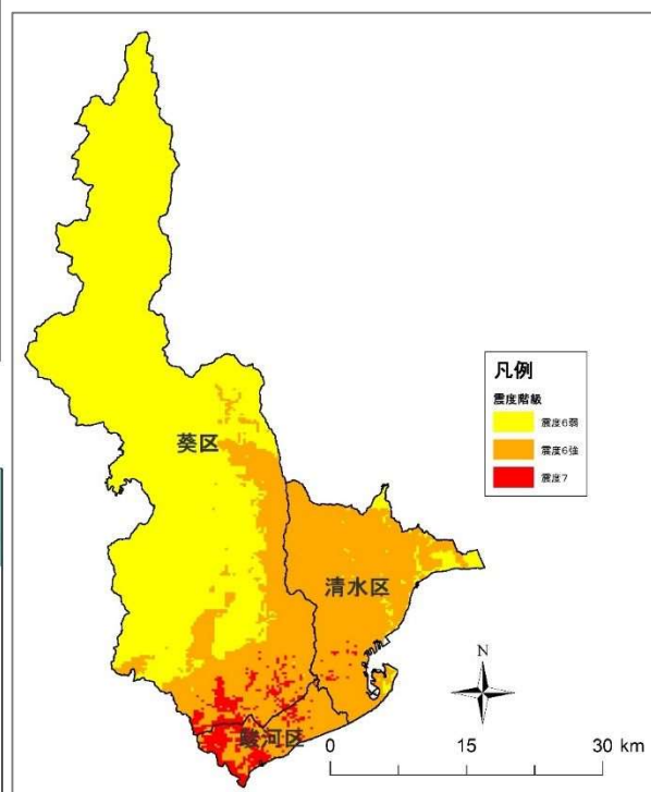
震度分布図（南海トラフ巨大地震 基本ケース）
