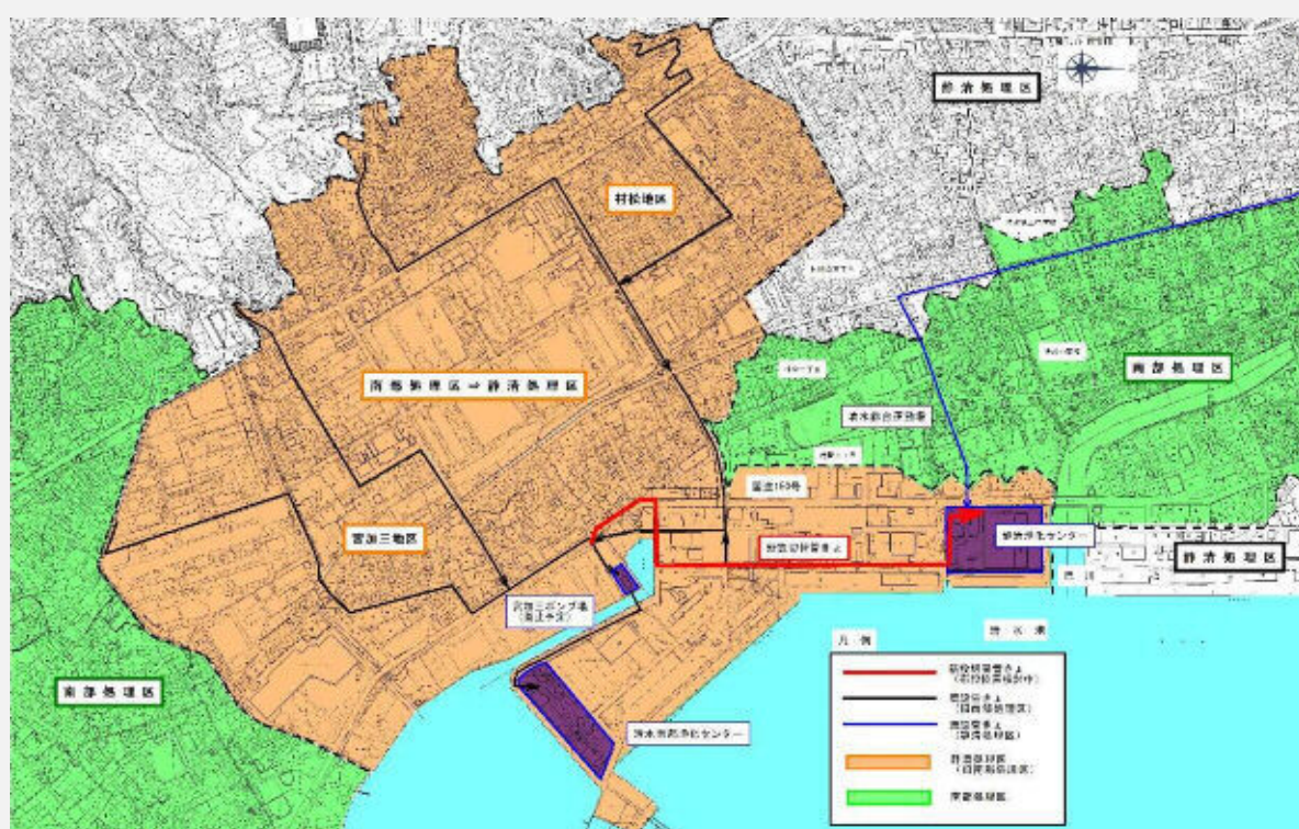
【処理区*切替工事概略図】
