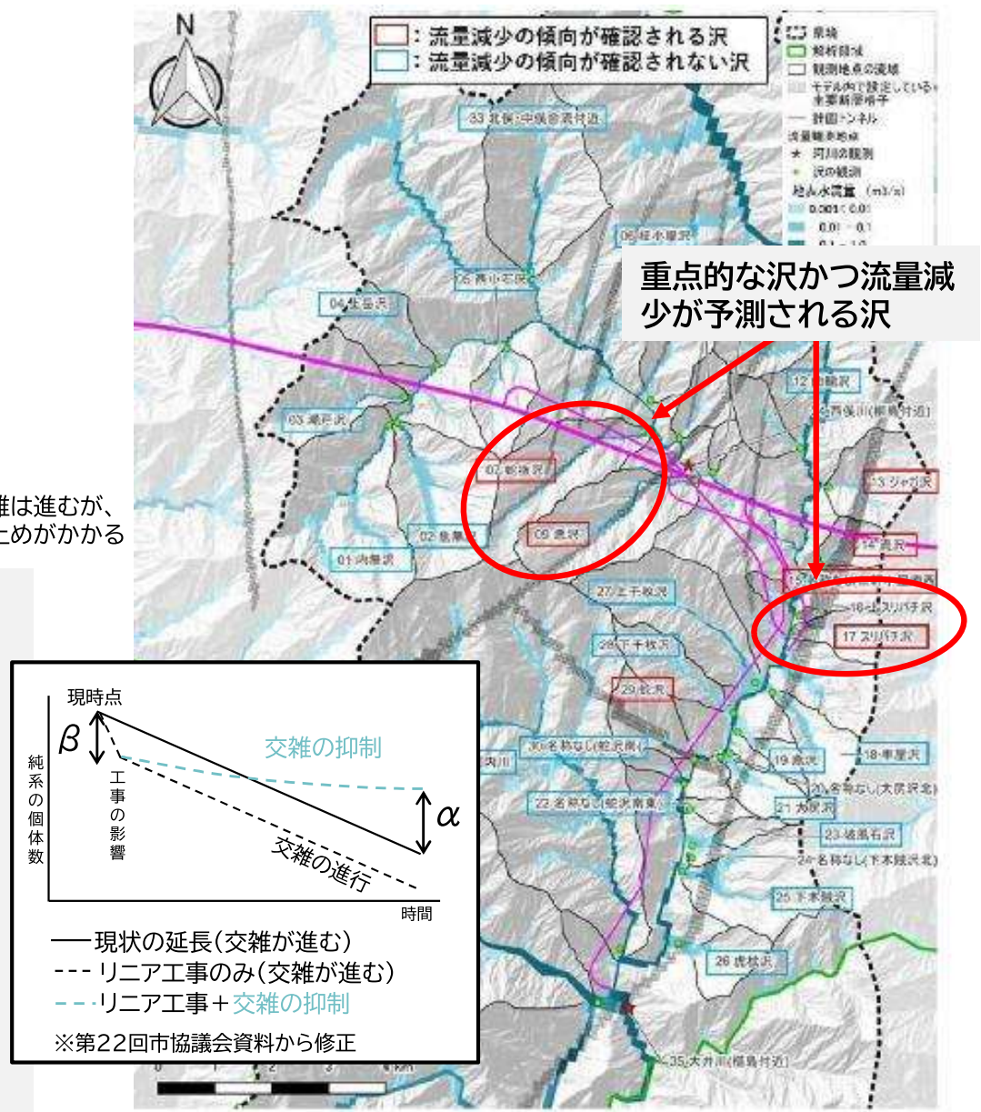
トンネル、主要な断層、沢流域の位置関係
