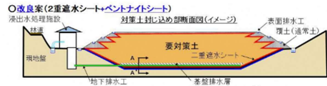
藤島における遮水構造計画図
