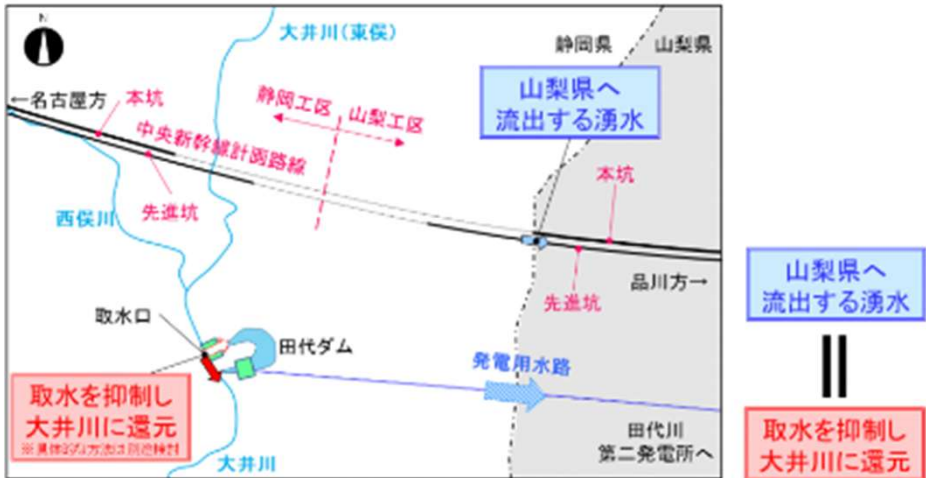
図3 工事の一定期間、発電のための取水を抑制し、大井川に還元する方策 出典:第12回静岡県地質構造・水資源部会専門部会(2023.3.20) 資料1 P14
