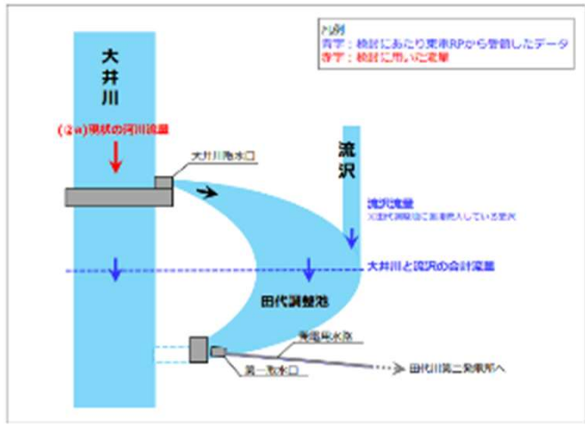
図4 田代ダムの取水イメージ 出典:第12回静岡県地質構造・水資源部会専門部会(2023.3.20) 資料1(別紙2) P29
