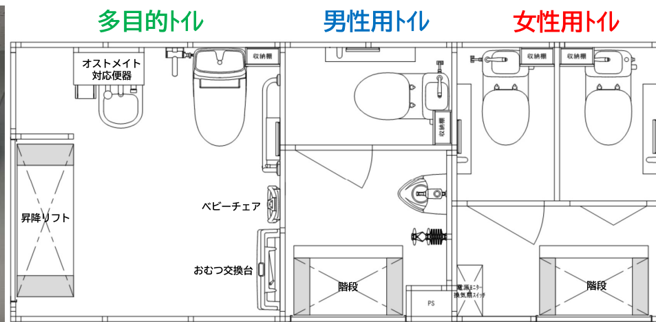
平面図
