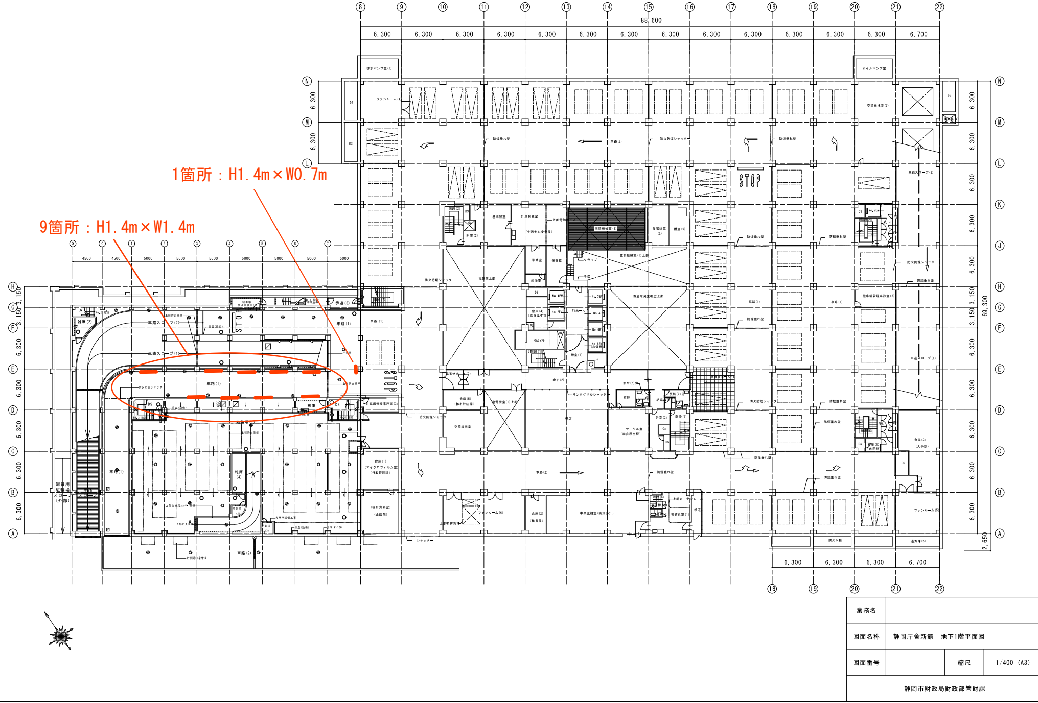
静岡庁舎新館地下 1 階駐車場 平面図
