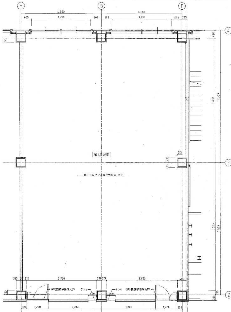
1階 第4練習場 平面詳細図 S 1:50
