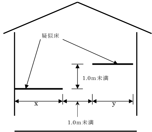
II (断面図)
