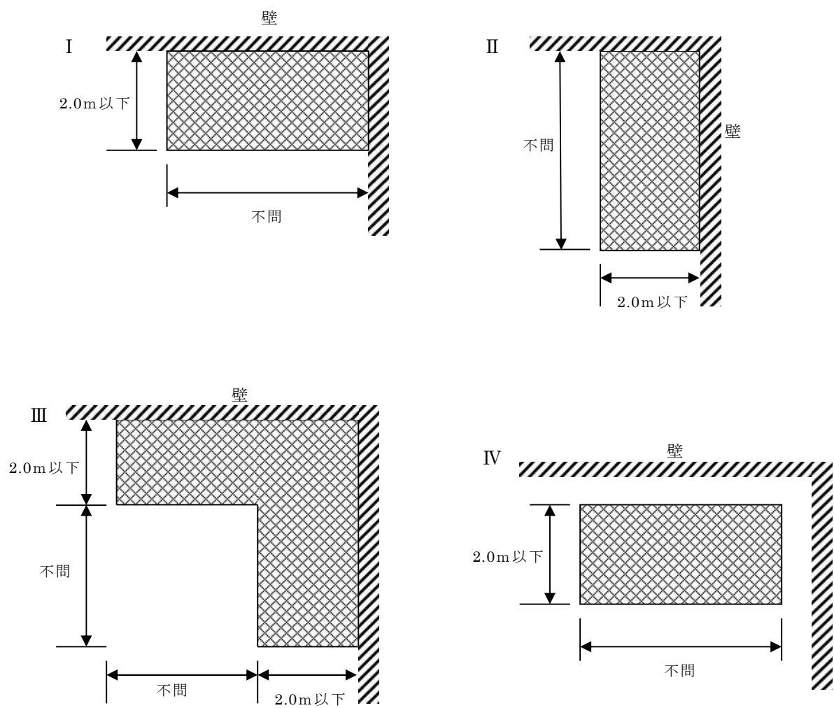
第 5 - 4 図 (平面図)
