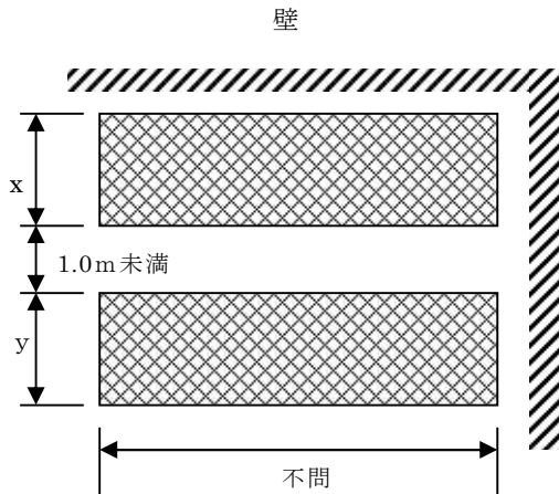
I (平面図)
