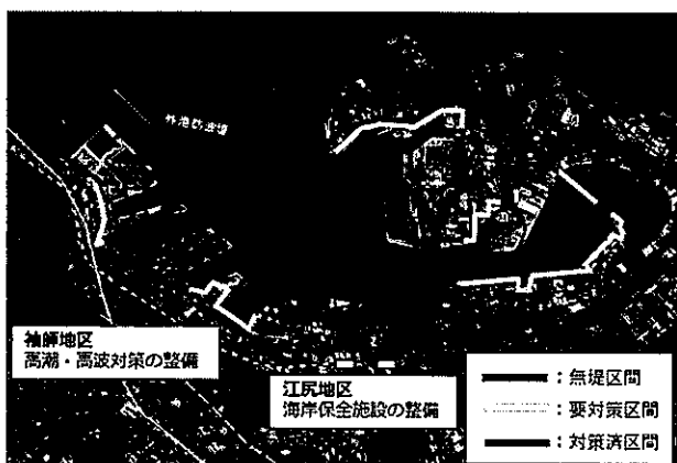
【清水港 平面図】
