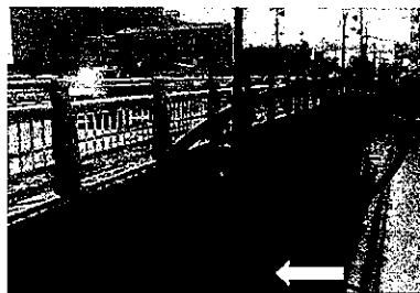
R4.9 台風 15 号時 漂流物が橋脚や橋桁に当たり、橋上に散乱
