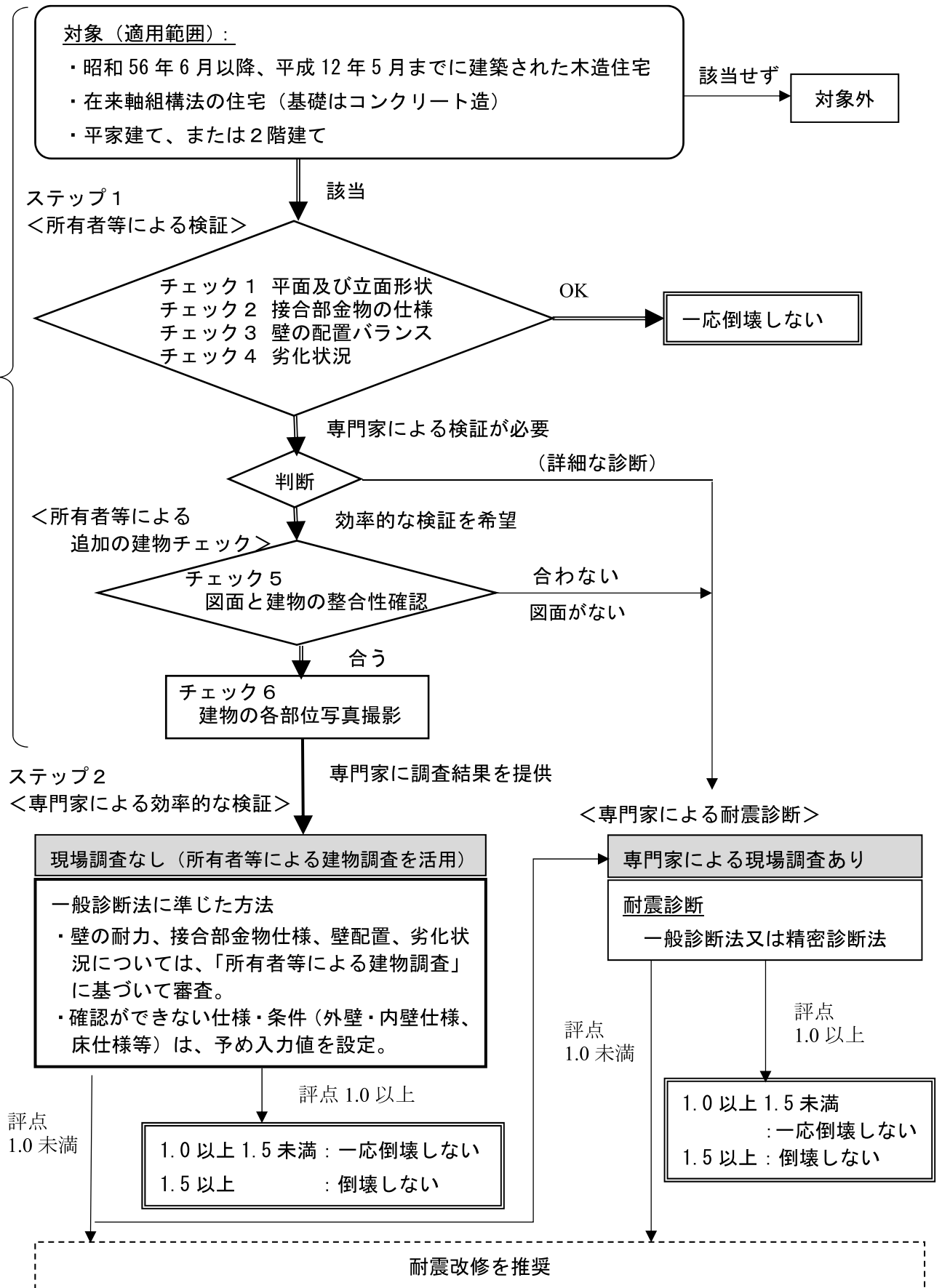
図 I.2 新耐震基準の木造住宅の耐震性能検証法のフロー図
