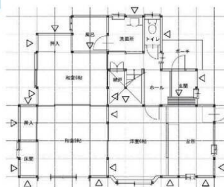
図面（平面図）の例
