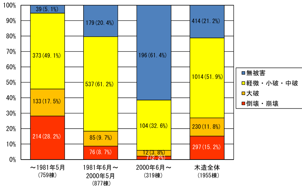
図2 学会悉皆調査結果による木造の建築時期別の被害状況
