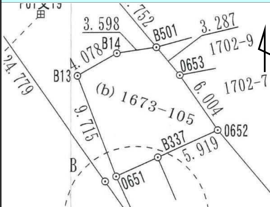
明細図
