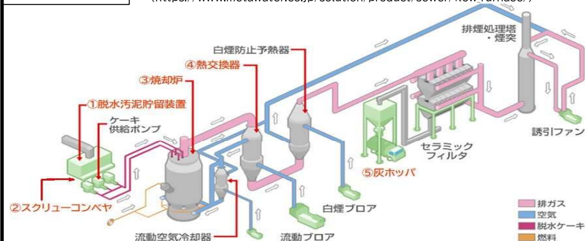
2号焼却炉フロー図
