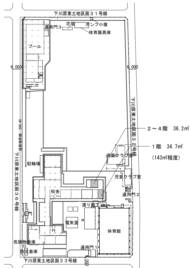
川原小学校 配置図 S=1:1500
