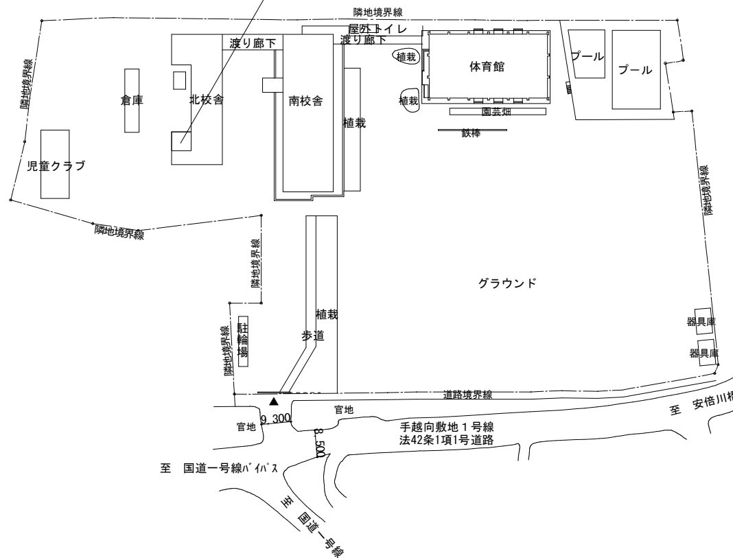
長田北小学校 配置図 S=1:1,500
