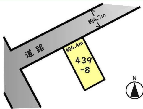
地形図
